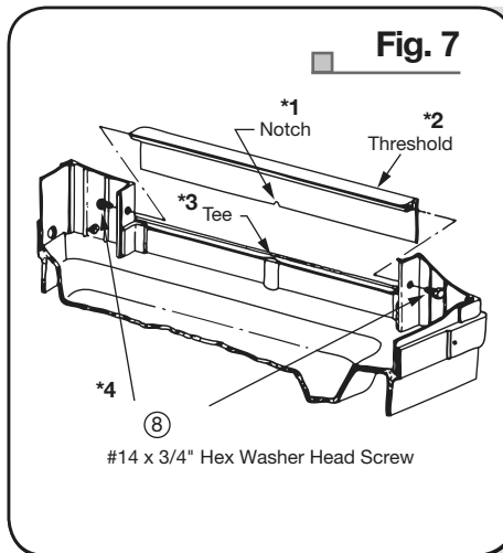
*1 Muesca *2 Ducha con umbral *3 Unión T *4 Tornillo de cabeza hexagonal con arandela del n.º 14 x 3/4" (19.05 mm)
