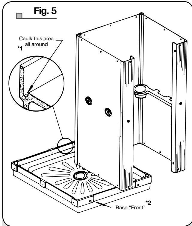
*1 Coloque masilla entorno a toda esta área. *2 Frente de la base
